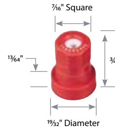
TXA ConeJet
